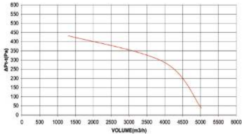
Ø250-1HP-1450RPM
